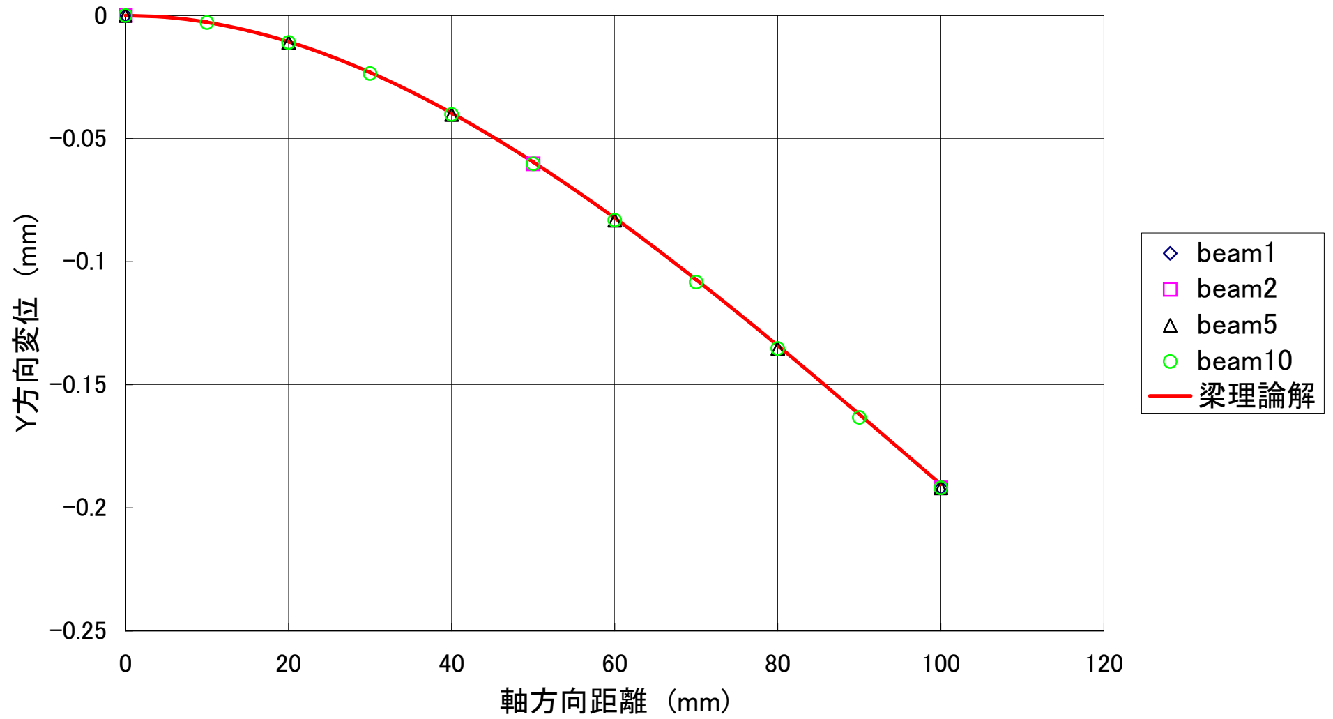
BEAM要素 變位
