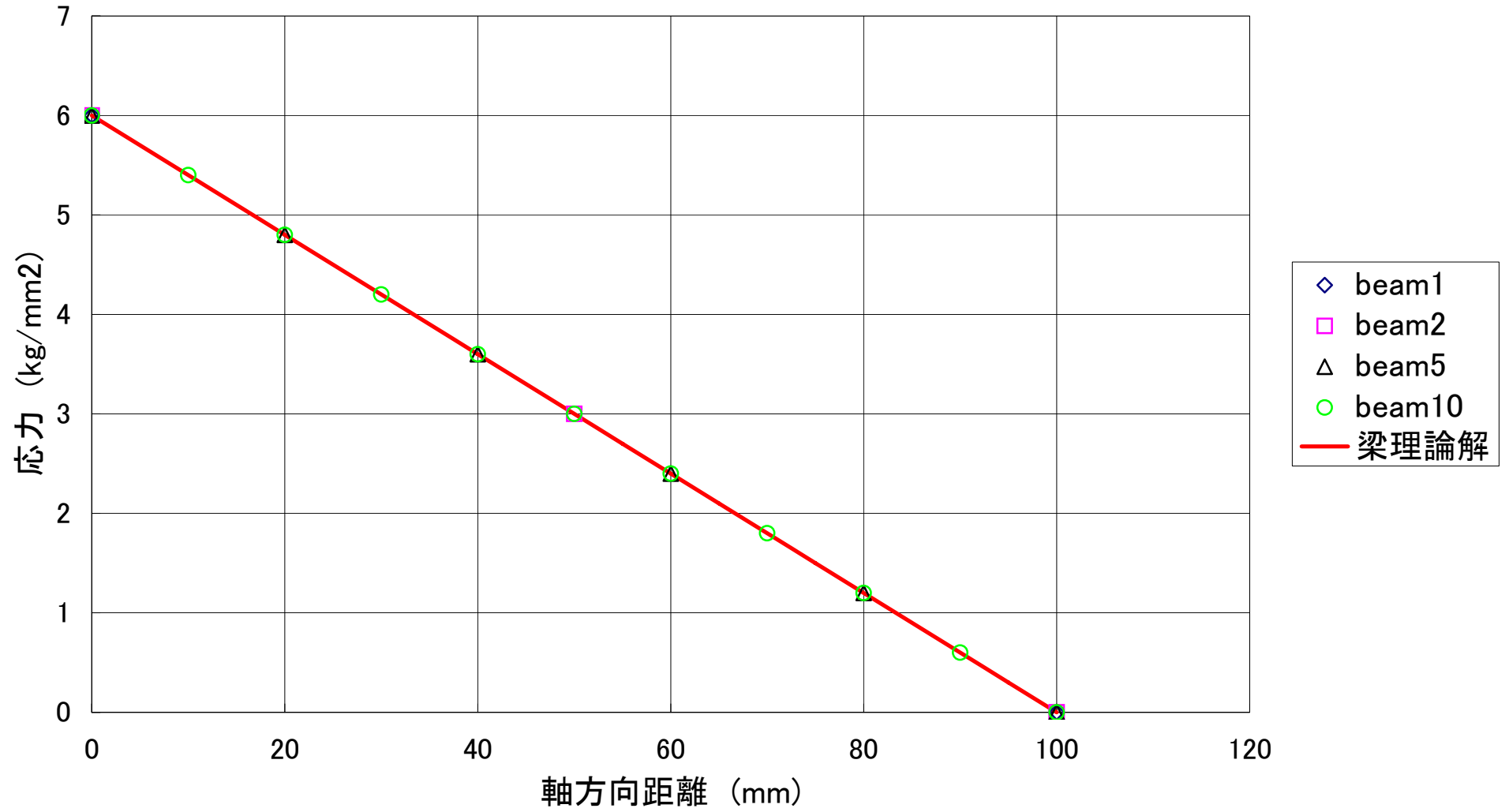
BEAM要素応力 最大主応力
